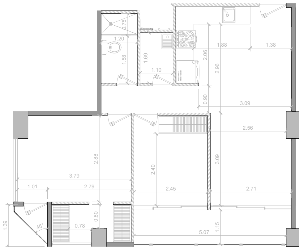
Planta Amoblada
